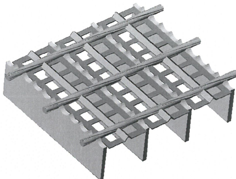
Rysunek A5. Kraty pomostowe i kraty stopni schodów TERMETAL, z bezpiecznymi oczkami SM (Security Mesh), z nacięciami typu „zęb piły” – widok
