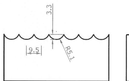
b) płaskownik nośny z nacięciami typu „ząb piły”
