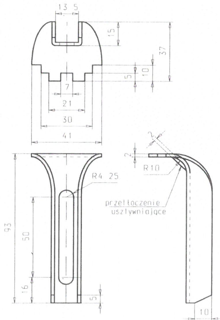
Rysunek A14. Uchwyt mocujący i spinający – część dolna
