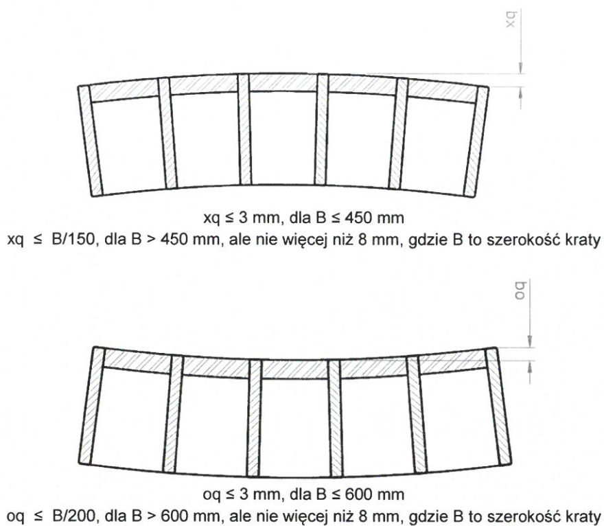
Rysunek A20. Dopuszczalne odchyłki kształtu – wygięcia wzdłuż prętów poprzecznych: wypukłość ( xq ) i wklęsłość ( oq )
