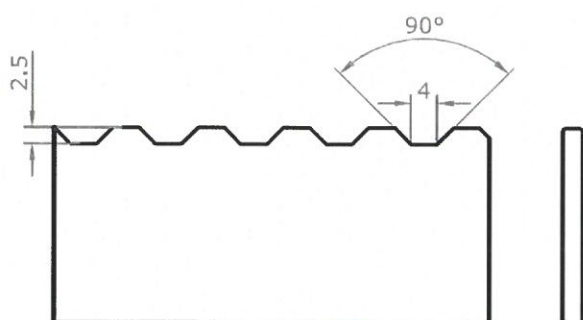
a) płaskownik nośny z nacięciami typu „trapez”
