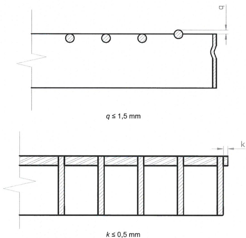
Rysunek A21. Dopuszczalne odchyłki kształtu – wystawanie prętów poprzecznych
